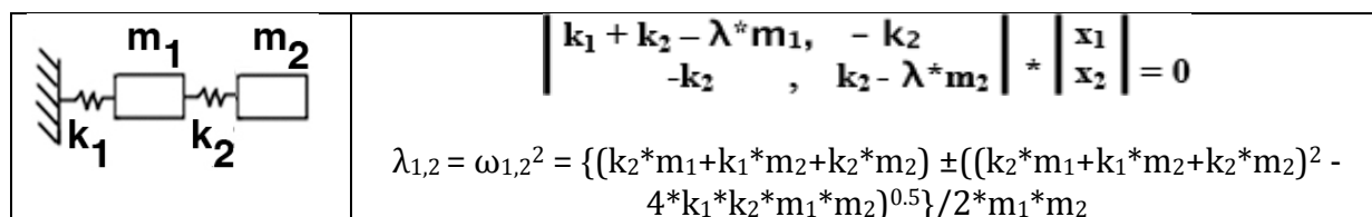
Рис. 4. Пример пружинно-массовой системы с двумя степенями свободы, массами m_1 и m_2 , жесткостью пружин k_1 и k_2 . Справа даны матричное уравнение для свободных колебаний объекта, а также выражения собственных значений \lambda_{1,2} .
